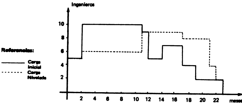
G. 16. Proyecto de Riego: nivelación de recursos por tanteo
