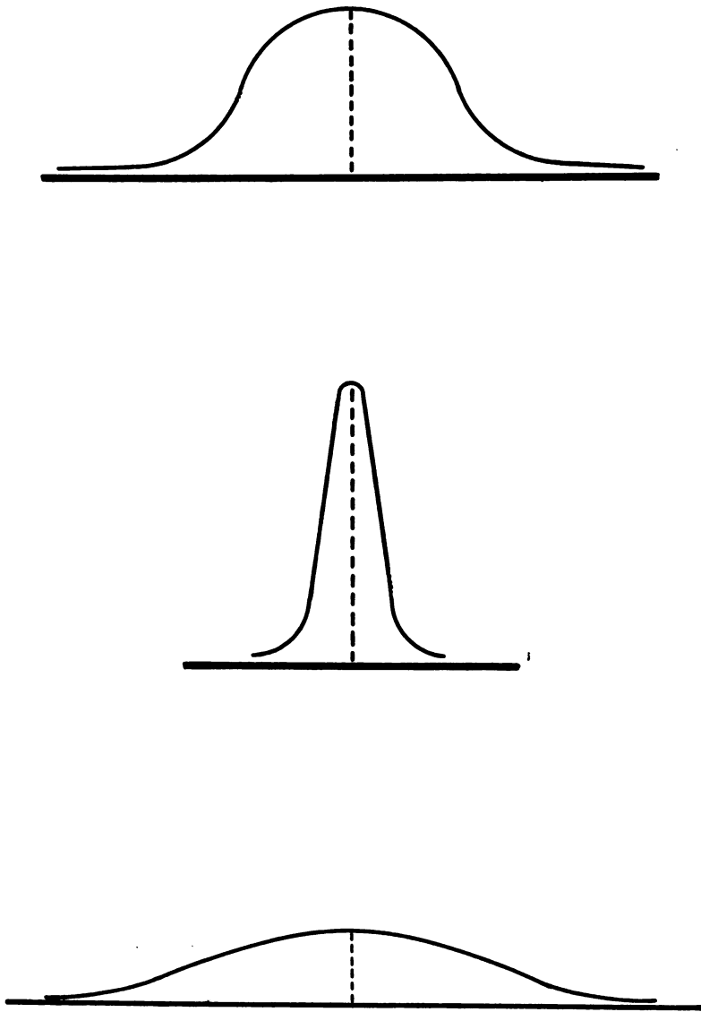
FIG. 18. Curvas normales con diferentes medias y desvíos.
