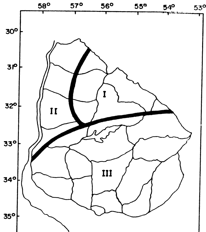
Figura 4. Regionalización agroclimática del cultivo de soja (Corsi, W. 1982)
