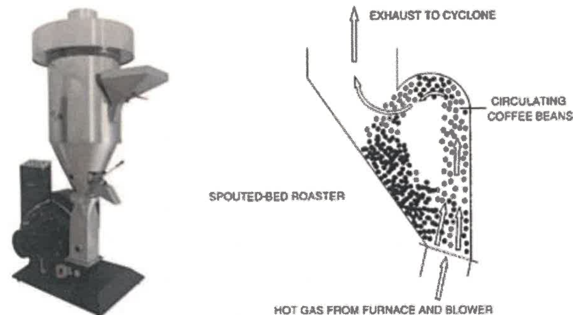
Tomado de www.boletinindustrial.com Figura 27. Tostador de lecho fluidizado
