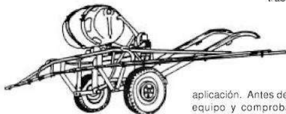
Figura 7. Pulverizador de herbicida de tracción animal.
