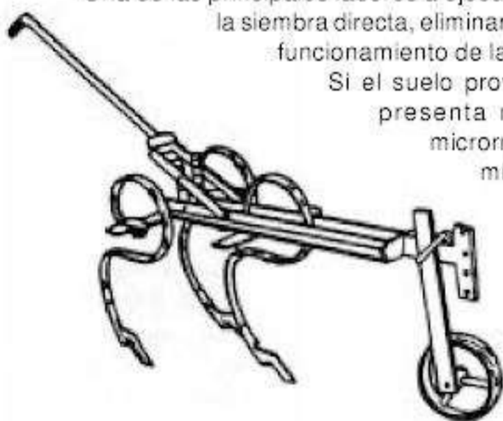
Figura 1. Arado cincel de tracción animal.
